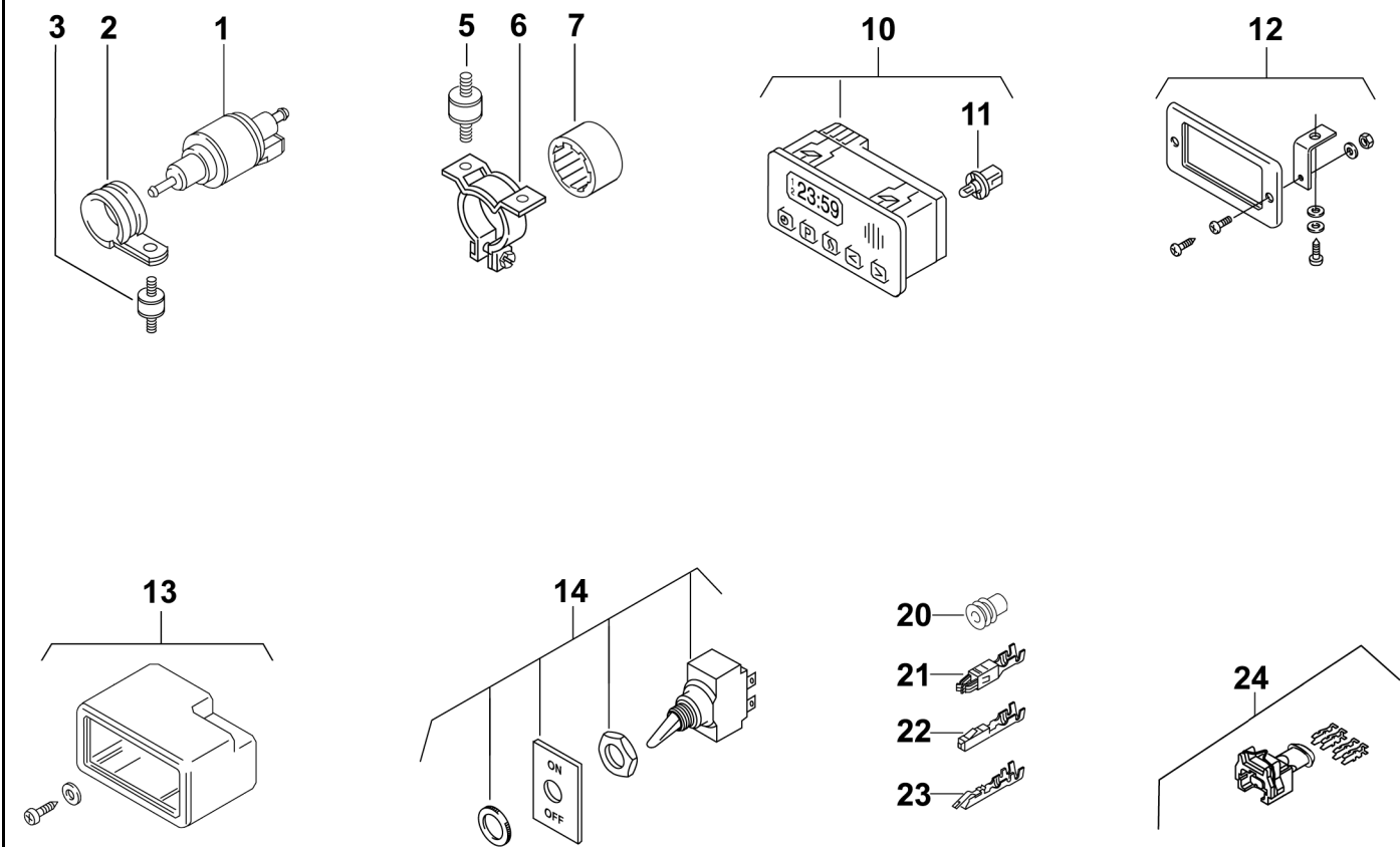
Thermo 50 (24 Volt, Diesel) - fig. 2
