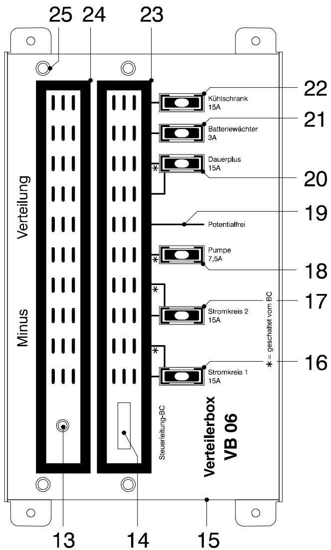
Bild 2: Verteilerbox VB 06
