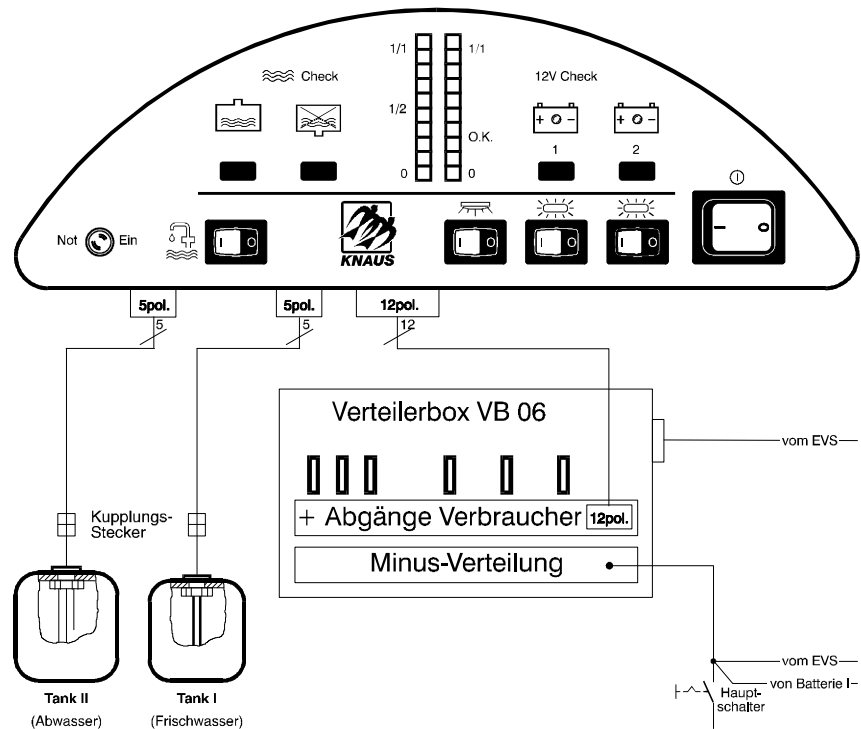
Bild 3: Anschlußplan BC 2000 und V-Box
